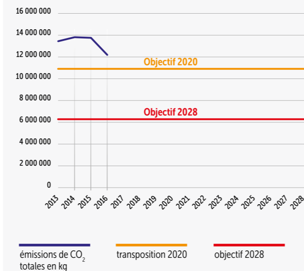
Évolution des émissions de CO 2 totales du patrimoine bâti NM/VdN à conditions climatiques standards
